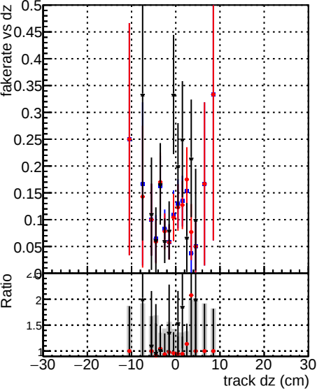
Fake rate vs dz DOM CKE test 1000evt DOM CKE test 1000evt DOM mkrFit test 1000evt
