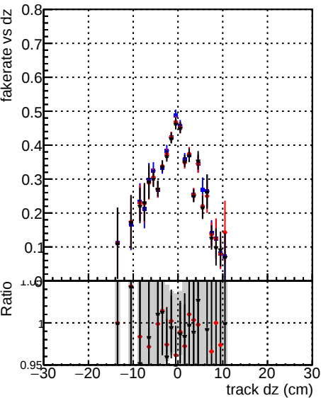
Fake rate vs dz Legend: DOM CKE fit 1000evt DOM CKE fit 1000evt DOM mkr fit 1000evt DOM mkr fit 1000evt
