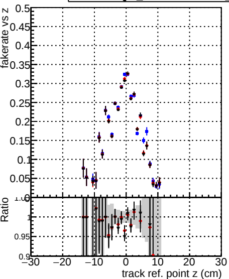
Fake rate vs v DOM_CKF-test_1000evt DOM_CKFREFit-test_1000evt DOM_mkFitREFit-test_1000evt
