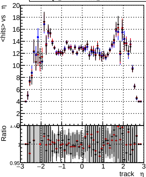
mean hit \eta — DQM_CKF-test_1000evt — DQM_CKFREFit-test_1000evt — DQM_mkFitREFit-test_1000evt
