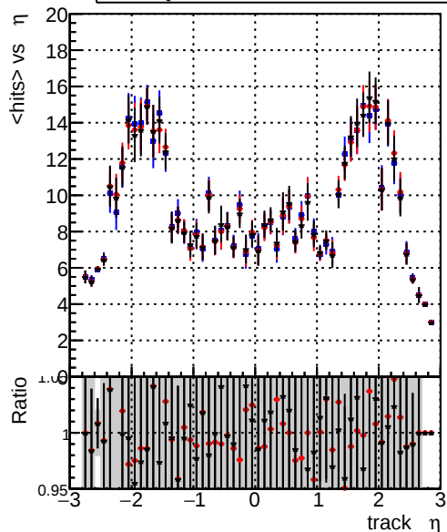
mean hits — DQM_CKF-test_1000evt — DQM_CKFFit-test_1000evt — DQM_mkFitREFit-test_1000evt
