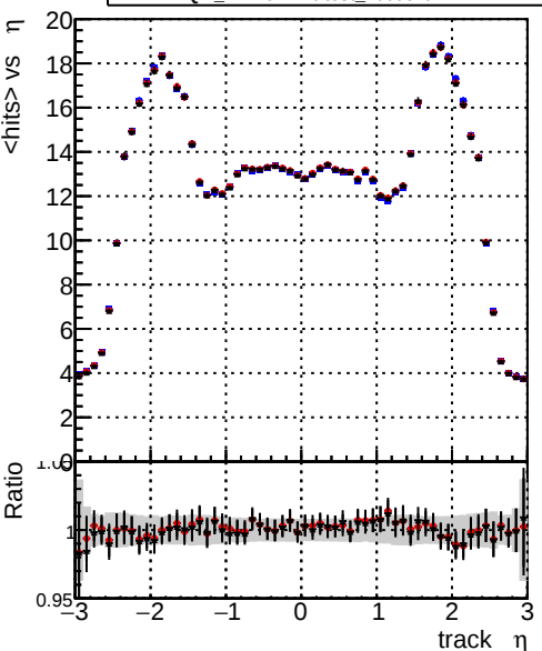
mean hits — DQM_CKF-test_1000evt — DQM_CKFREFit-test_1000evt — DQM_mkFitREFit-test_1000evt
