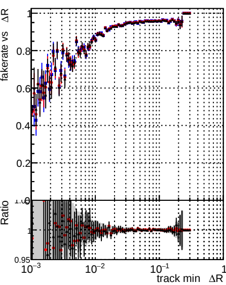
—•— DQM_CKF-test_1000evt —•— DQM_CKFREFit-test_1000evt —•— DQM_mkFitREFit-test_1000evt
