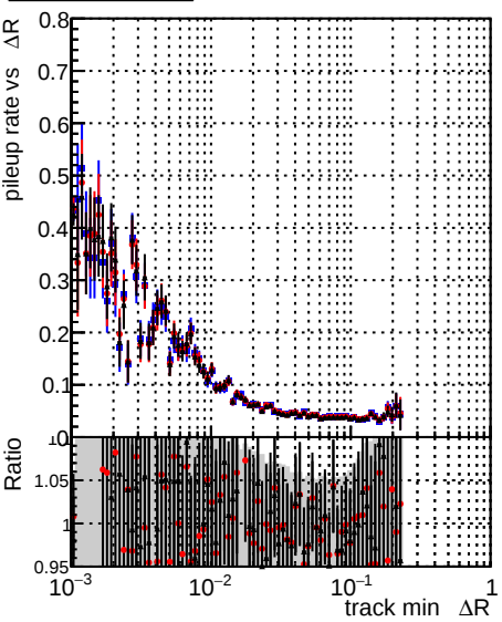
—•— DQM_CKF-test_1000evt —•— DQM_CKFREFit-test_1000evt —•— DQM_mkFitREFit-test_1000evt
