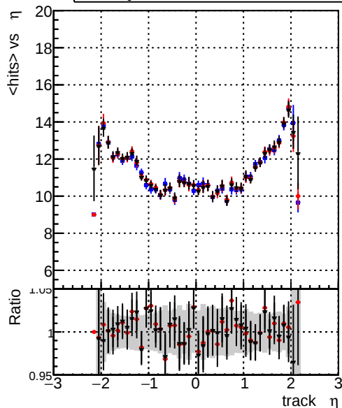
mean hits vs \eta — DQM_CKF-test_1000evt — DQM_CKFFit-test_1000evt — DQM_mkFitREFit-test_1000evt
