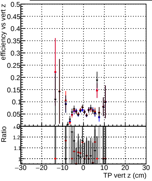
Efficiency vs TP vert z (cm) Legend: DQM_CKF-test_1000evt (blue circles) DQM_CKFREFit-test_1000evt (red circles) DQM_mkFitREFit-test_1000evt (black circles)
