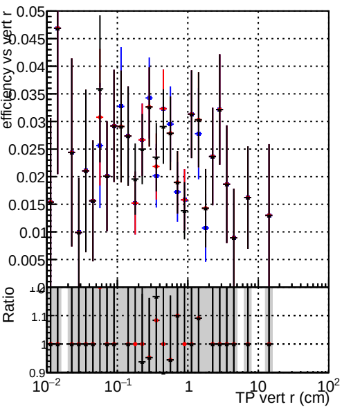
Efficiency vs TP vert r (cm) Legend: DQM_CKF-test_1000evt DQM_CKFREFit-test_1000evt DQM_mkFitREFit-test_1000evt
