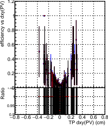
Efficiency vs Dxy(PV) DQM_CKF-test_1000evt DQM_CKFREFit-test_1000evt DQM_mkFitREFit-test_1000evt
