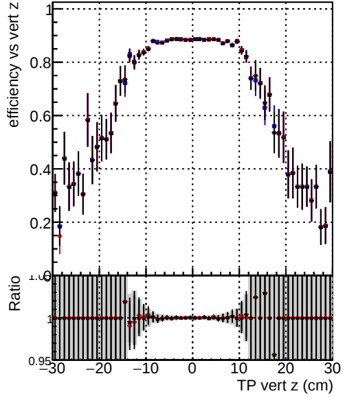
Efficiency vs. sim PV z — DQM_CKF-test_1000evt — DQM_CKFitFit-test_1000evt — DQM_mkFitFit-test_1000evt
