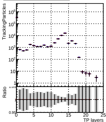
N of sim → DQM_mkFitREFit-test_1000evt
