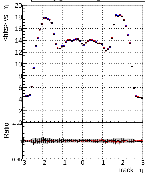
mean hits — DQM_CKF-test_1000evt — DQM_CKFREFit-test_1000evt — DQM_mkFitREFit-test_1000evt
