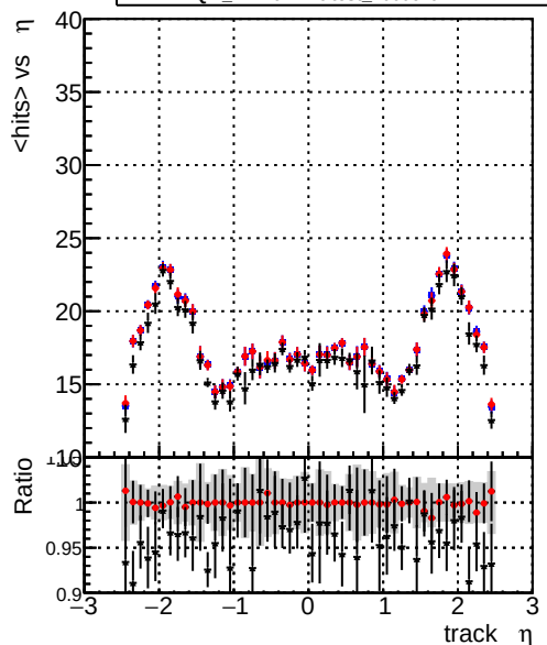
mean hits vs \eta — DQM_CKF-test_1000evt — DQM_CKFREFit-test_1000evt — DQM_mkFitREFit-test_1000evt
