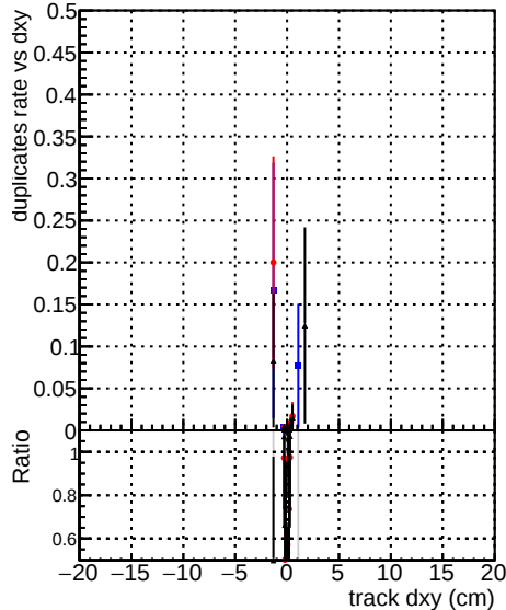
ttbar-phase1-newgeom
