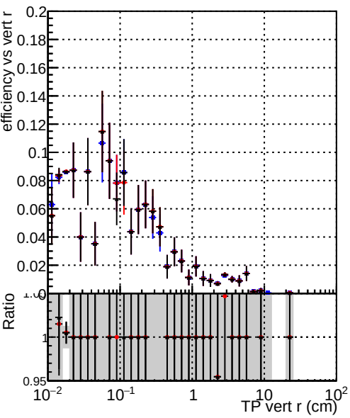
Efficiency vs TP vert r (cm) Legend: DQM_CKFFit_1000evt DQM_CKFREFitOLD_1000evt DQM_MkFitREFitOLD_1000evt
