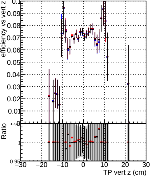
Efficiency vs TP vert z (cm) Legend: DQM_CKFFit_1000evt DQM_CKFREFitOLD_1000evt DQM_MkFitREFitOLD_1000evt
