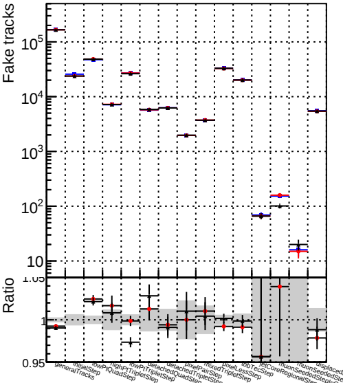
Number —●— DQM_CKFREFitOLD_1000evt —▲— DQM_MkFitREFitOLD_1000evt
