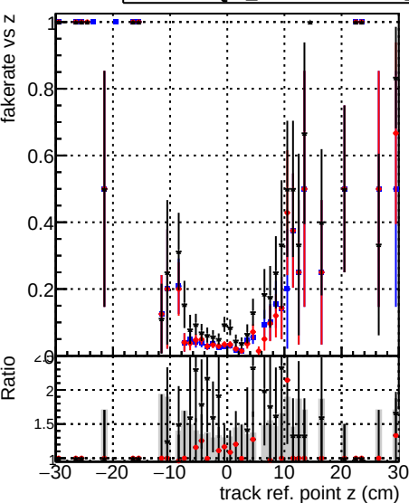
Fake rate vs DOM CKFFit 1000evt DOM CKFREFitOLD 1000evt DOM MkFitREFitOLD 1000evt
