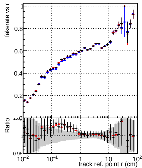
Fake rate vs DOM CKFFit 1000evt DOM CKFREFitOLD 1000evt DOM MkFitREFitOLD 1000evt
