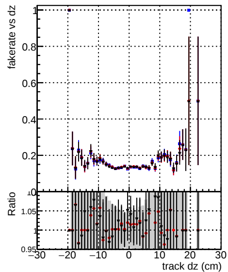
Fake rate vs d DOM CKFit 1000evt DOM CKREFitOLD 1000evt DOM MKFitREFitOLD 1000evt
