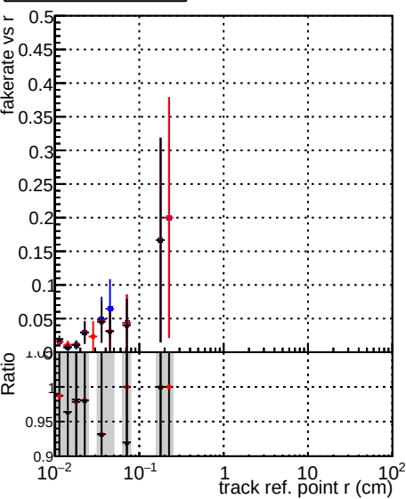
Fake rate vs vertpos DOM CKFFit 1000evt DOM CKFREFitOLD 1000evt DOM MkFitREFitOLD 1000evt
