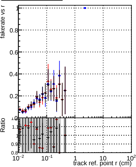
Fake rate vs v DOM_CKFFit_1000evt DOM_CKFFitOLD_1000evt DOM_MkFitREFitOLD_1000evt
