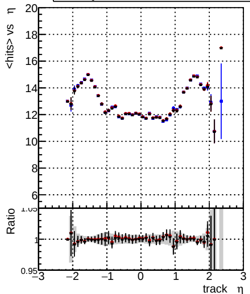
mean hits vs \eta — DQM_CKFFit_1000evt — DQM_CKFFitOLD_1000evt — DQM_MkFitREFitOLD_1000evt
