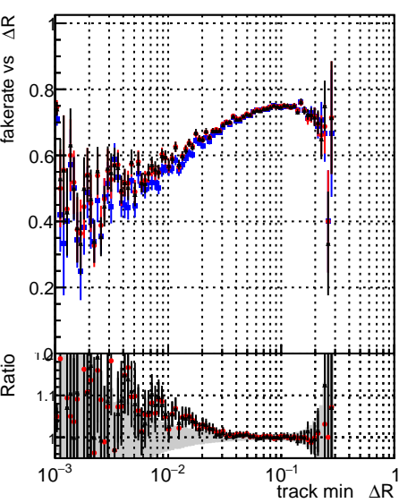
■ DQM_CKFFit_1000evt ● DQM_CKFREFitOLD_1000evt ▲ DQM_MkFitREFitOLD_1000evt
