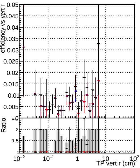
Efficiency vs TP vert r (cm) Legend: DQM_CKFFit_1000evt DQM_CKFFitOLD_1000evt DQM_MkFitREFitOLD_1000evt
