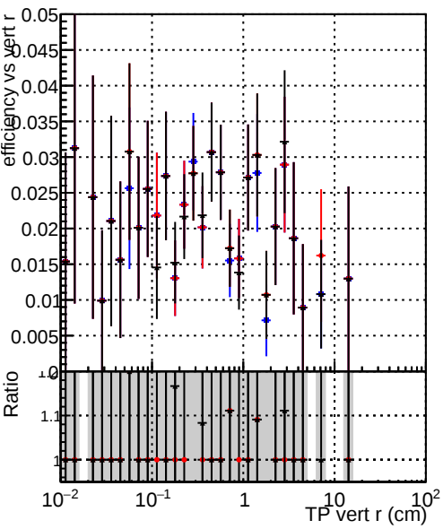
Efficiency vs vertpos Legend: DQM_CKFFit_1000evt DQM_CKFREFitOLD_1000evt DQM_MkFitREFitOLD_1000evt
