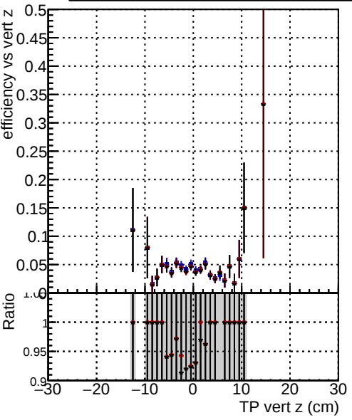
Efficiency vs TP vert z (cm) Legend: DQM_CKFFit_1000evt (blue) DQM_CKFREFitOLD_1000evt (red) DQM_MkFitREFitOLD_1000evt (black)
