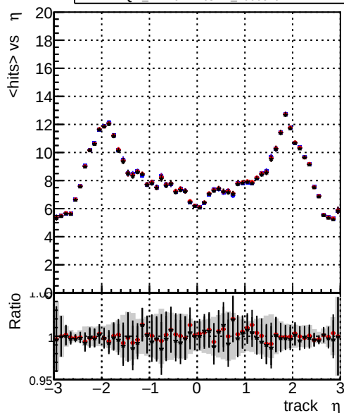
mean hits vs \eta — DQM_CKFFit_1000evt — DQM_CKFFitOLD_1000evt — DQM_MkFitREFitOLD_1000evt
