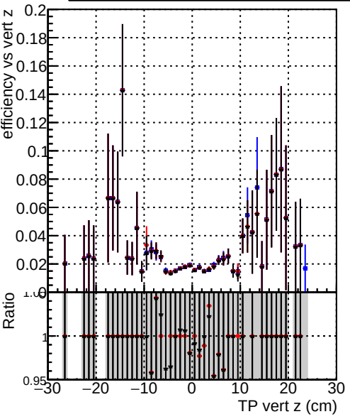
Efficiency vs TP vert z (cm) Legend: DQM_CKFFit_1000evt (blue) DQM_CKFREFit_1000evt (red) DQM_MkFitREFit_1000evt (black)
