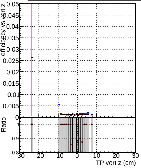
Efficiency vs vertpos Legend: DQM_CKFFit_1000evt DQM_CKFREFit_1000evt DQM_MkFitREFit_1000evt
