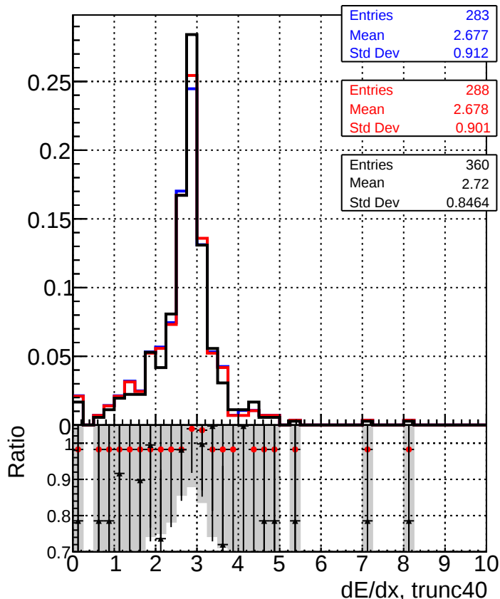
—■— DQM_CKFFit_1000evt —●— DQM_CKFREFit_1000evt —▲— DQM_MkFitREFit_1000evt
