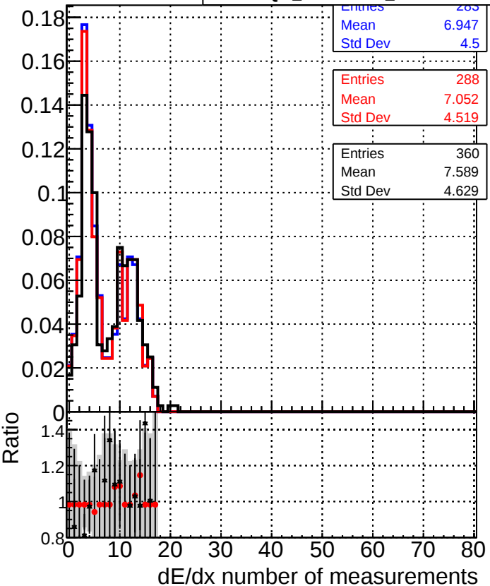
—■— DQM_CKFFit_1000evt —●— DQM_CKFREFit_1000evt —▲— DQM_MkFitREFit_1000evt
