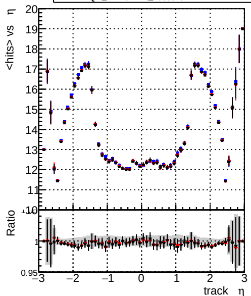
mean hits vs \eta — DQM_CKFFit_1000evt — DQM_CKFREFit_1000evt — DQM_MkFitREFit_1000evt
