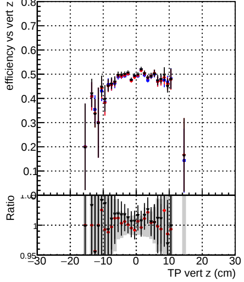
Efficiency vs. sim PV z —●— DQM_CKFFit_1000evt —●— DQM_CKFREFit_1000evt —●— DQM_MkFitREFit_1000evt
