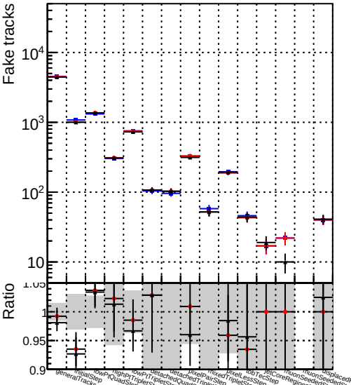
Number —●— DQM_CKFFit_1000evt —★— DOM_MkFitREFit_1000evt
