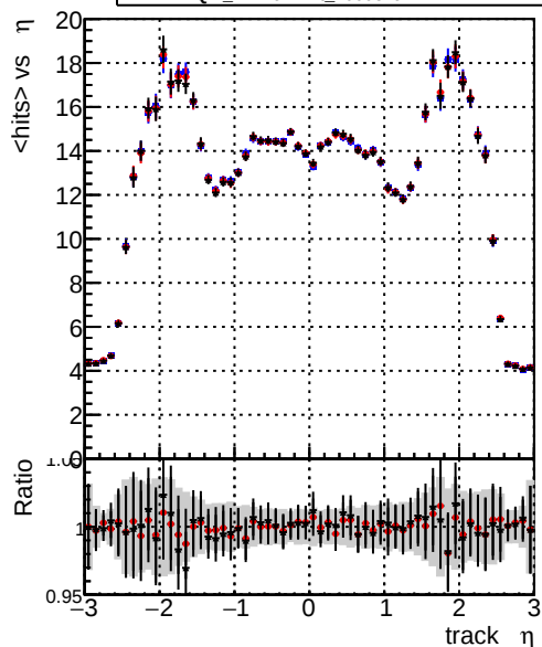
mean hit — DQM_CKFFit_1000evt — DQM_CKFREFit_1000evt — DQM_MkFitREFit_1000evt
