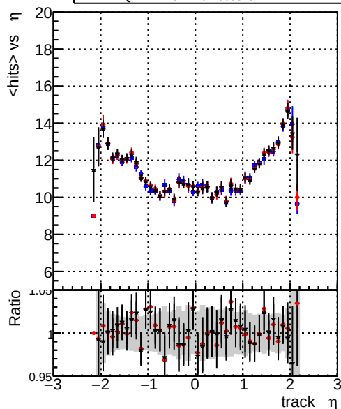
mean hits vs \eta — DQM_CKFFit_1000evt — DQM_CKFREFit_1000evt — DQM_MkFitREFit_1000evt
