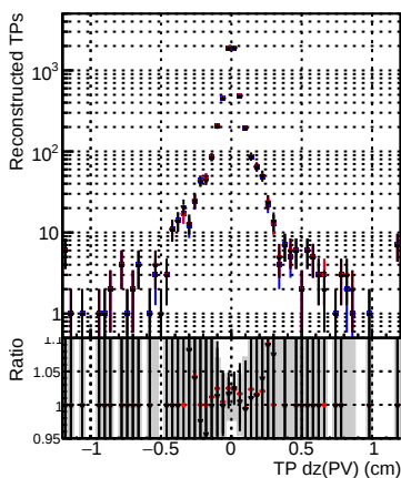
N of associated tracks (simToReco) vs dz(PV) 0 1 1 1 2 1 3 1 4 1 5 1 6 1 7 1 8 1 9 1 10 1 11 1 12 1 13 1 14 1 15 1 16 1 17 1 18 1 19 1 20 1 21 1 22 1 23 1 24 1 25 1 26 1 27 1 28 1 29 1 30 1 31 1 32 1 33 1 34 1 35 1 36 1 37 1 38 1 39 1 40 1 41 1 42 1 43 1 44 1 45 1 46 1 47 1 48 1 49 1 50 1 51 1 52 1 53 1 54 1 55 1 56 1 57 1 58 1 59 1 60 1 61 1 62 1 63 1 64 1 65 1 66 1 67 1 68 1 69 1 70 1 71 1 72 1 73 1 74 1 75 1 76 1 77 1 78 1 79 1 80 1 81 1 82 1 83 1 84 1 85 1 86 1 87 1 88 1 89 1 90 1 91 1 92 1 93 1 94 1 95 1 96 1 97 1 98 1 99 1 100 1 101 1 102 1 103 1 104 1 105 1 106 1 107 1 108 1 109 1 110 1 111 1 112 1 113 1 114 1 115 1 116 1 117 1 118 1 119 1 120 1 121 1 122 1 123 1 124 1 125 1 126 1 127 1 128 1 129 1 130 1 131 1 132 1 133 1 134 1 135 1 136 1 137 1 138 1 139 1 140 1 141 1 142 1 143 1 144 1 145 1 146 1 147 1 148 1 149 1 150 1 151 1 152 1 153 1 154 1 155 1 156 1 157 1 158 1 159 1 160 1 161 1 162 1 163 1 164 1 165 1 166 1 167 1 168 1 169 1 170 1 171 1 172 1 173 1 174 1 175 1 176 1 177 1 178 1 179 1 180 1 </
