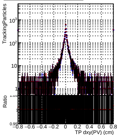
N of sim → DQM_MkFitREFit_1000e
