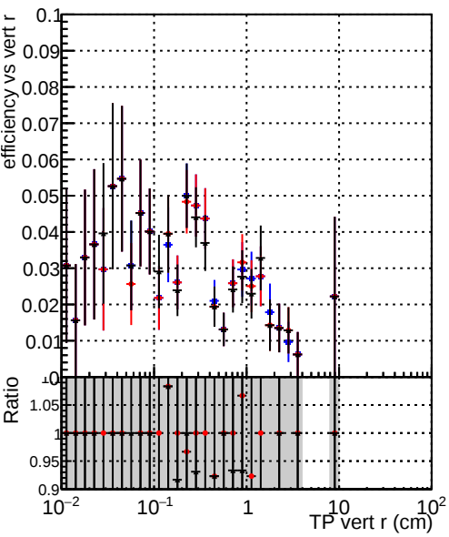
Efficiency vs TP vert r (cm) Legend: DQM_CKFFit_1000evt (blue) DQM_CKFREFit_1000evt (red) DQM_MkFitREFit_1000evt (black)
