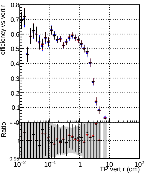
Efficiency vs TP vert r (cm) Legend: DQM_CKFFit_1000evt DQM_CKFREFit_1000evt DQM_MkFitREFit_1000evt
