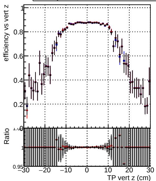
Efficiency vs vert z — DQM_CKFFit_1000evt — DQM_CKFFit_1000evt — DQM_MkFitREFit_1000evt
