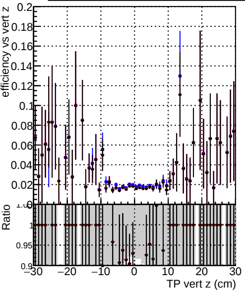
Efficiency vs TP vert z (cm) plot Legend: DQM_original_originalvector_1000evt DQM_fit_cpeOK_SORTRZ2_TESTOUTLIER5_1000evt DQM_fit_cpeOK_SORTRZ2_TESTOUTLIER6_1000evt
