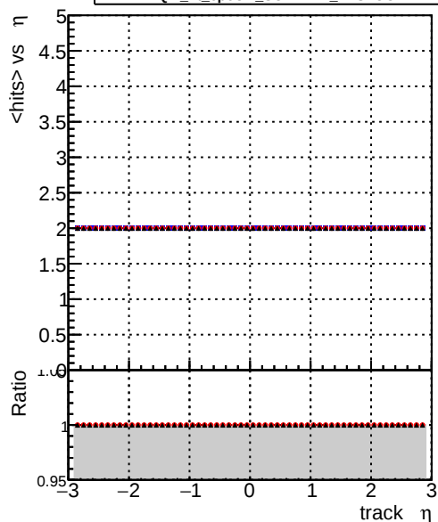
mean hits vs \eta — DQM_original_originalvector_1000evt — DQM_fit_cpeOK_SORTRZ2_TESTOUTLIER5_1000evt — DQM_fit_cpeOK_SORTRZ2_TESTOUTLIER6_1000evt
