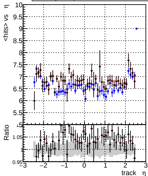
mean hits DQM_original_originalvector_1000evt DQM_fit_cpeOK_SORTRZ2_TESTOUTLIER5_1000evt DQM_fit_cpeOK_SORTRZ2_TESTOUTLIER6_1000evt
