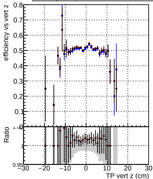
Efficiency vs vert z — DQM_originalvector_1000evt — DQM_fit_cpeOK_SORTRZ2_TESTOUTLIER5_1000evt — DQM_fit_cpeOK_SORTRZ2_TESTOUTLIER6_1000evt
