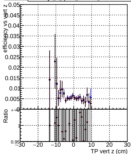
Efficiency vs. TP vert z (cm) —●— DQM_original_originalvector_1000evt —●— DQM_fit_cpeOK_SORTRZ2_TESTOUTLIER5_1000evt —●— DQM_fit_cpeOK_SORTRZ2_TESTOUTLIER6_1000evt
