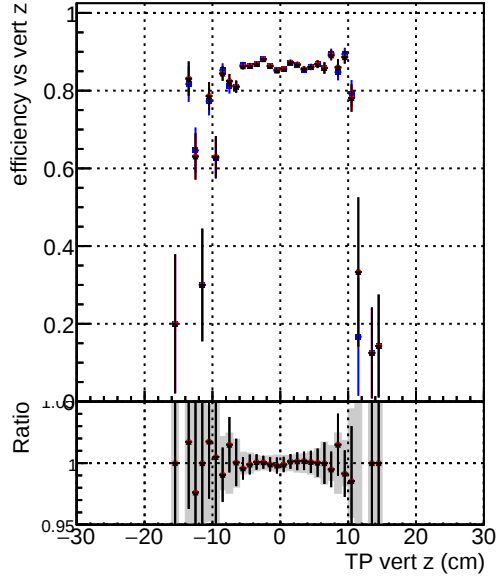
Efficiency vs TP vert z —●— DQM_original_originalvector_1000evt —●— DQM_fit_cpeOK_SORTRZ2_TESTOUTLIER5_1000evt —●— DQM_fit_cpeOK_SORTRZ2_TESTOUTLIER6_1000evt
