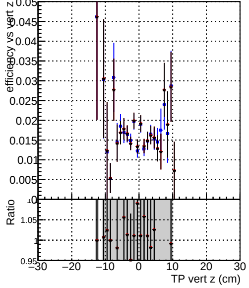
Efficiency vs. sim PV z DQM_fit_cpeOK_SORTRZ2_TESTOUTLIER5_1000evt DQM_fit_cpeOK_SORTRZ2_TESTOUTLIER6_1000evt DQM_originalvector_1000evt
