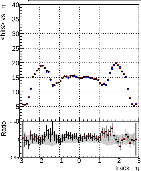
mean hits vs \eta — DQM_fit_cpeOK_SORTRZ2_TESTOUTLIER5_1000evt — DQM_fit_cpeOK_SORTRZ2_TESTOUTLIER6_1000evt
